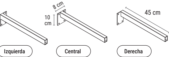
Soporte metálico lacado epoxi color blanco White epoxy lacquered metal support · Support métallique laqué époxy blanc · Supporto in metallo laccato epossidico bianco · Weiß lackierter Epoxidmetallträger
